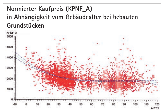
Abb. 8: Darstellung funktionaler Zusammenhänge
