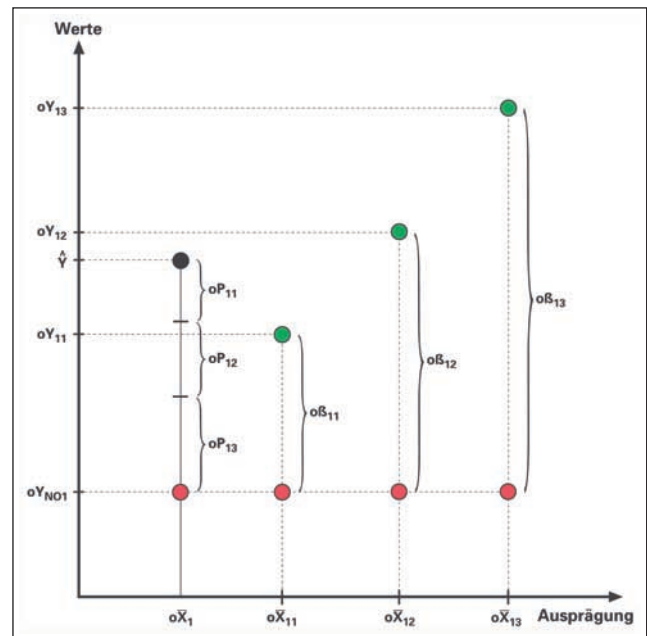
Abb. 4: Prinzip zur Auflösung ordinalskalierteter Ausprägungen
