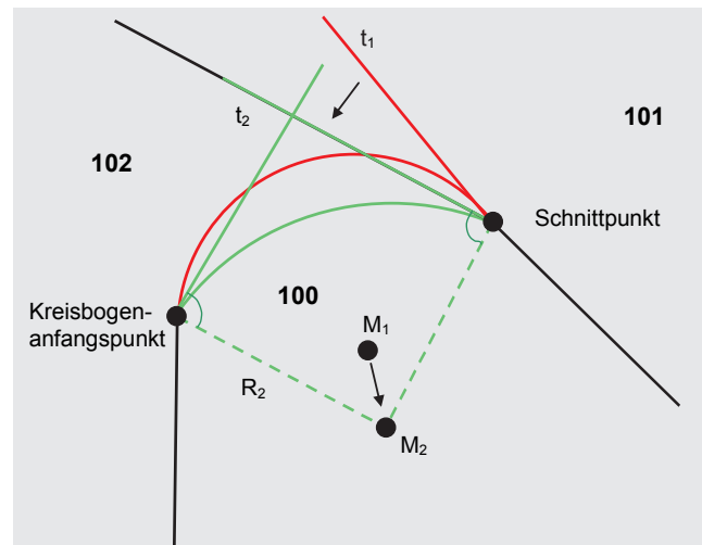
Abb. 5: Ableitung neuer Kreisbogenparameter durch Herstellung der Identität von Kreisbogentangente und abgehender Flurstücksgrenze
