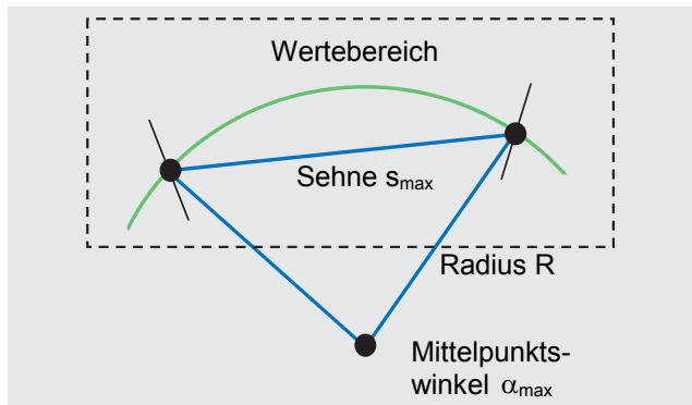
Abb. 12: Bestimmung des Wertebereichs zu den Parametern Radius R , Sehne s_{\max} und/oder Mittelpunktswinkel \alpha_{\max}
