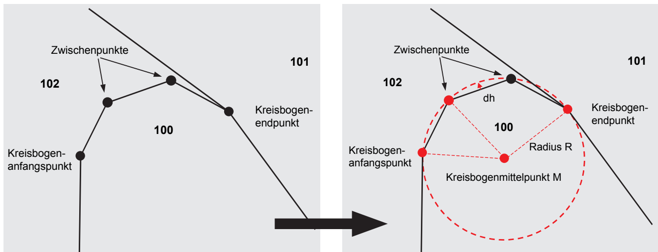
Abb. 11: Rekonstruktion der Kreisbogenparameter aus einem linearisierten Kreisbogen
