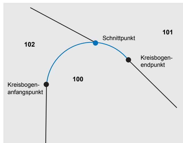
Abb. 8: Prinzipische Skizze Variante 2 (2) »Schnittbildung und Bereinigung Grenzverlauf«/Bereinigung durch Löschen der schneidenden Sekante
