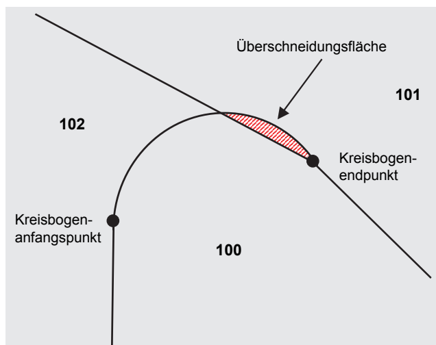
Abb. 3: Prinzipskizze zur Flächenüberschneidung bei ALK-Definitionsgeometrien mit Kreisbögen
