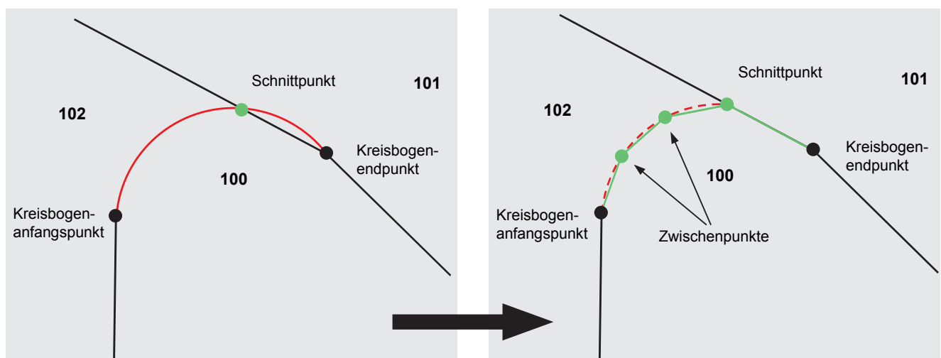
Abb. 10: Prinzipische Skizze Variante 3 (2) »Kreisbogenlinearisierung« mit Schnittpunktbildung und Linearisierung des Kreisbogens
