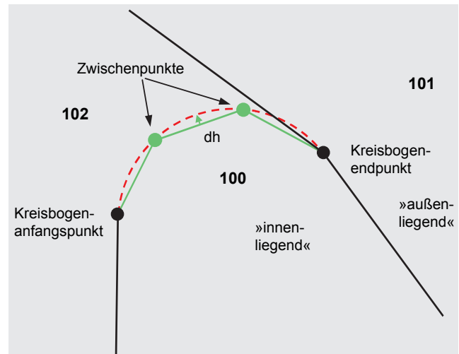
Abb. 9: Prinzipische Skizze Variante 3 (1) »Kreisbogenlinearisierung«
