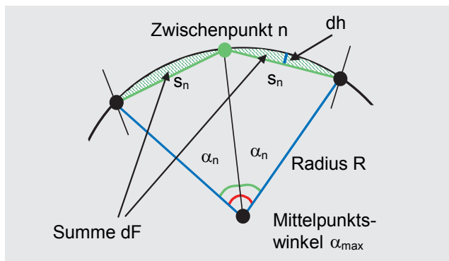
Abb. 13: Bestimmung der Anzahl zusätzlicher Stützpunkte und der Flächendifferenz bei Vorgabe des Wertebereichs und der Pfeilhöhe dh
