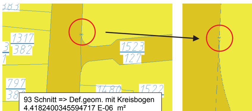
Abb. 2: Beispiel für eine Flächenüberschneidung bei Kreisbogengeometrie und abgehender Flurstücksgrenze in der Folie 001 (Flurstücke) der Automatisierten Liegenschaftskarte (ALK)
