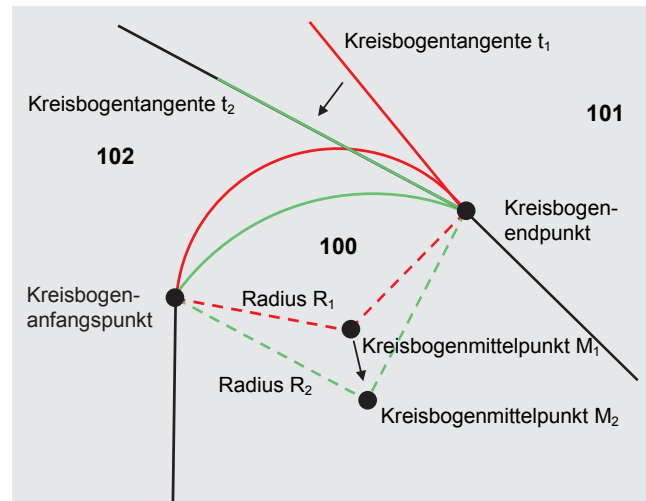
Abb. 4: Prinzipskizze zur Variante 1 »Variation Kreisbogenparameter«
